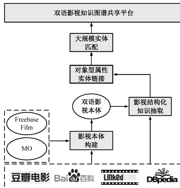
图 1 双语影视知识图谱构建流程图 Fig. 1 Pipeline of the BMKG
