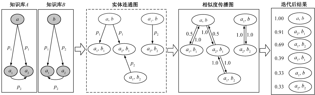
图 2 基于 Similarity Flooding 的实体匹配算法示意图 [9]
